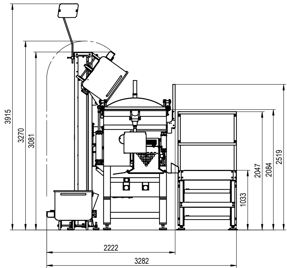
ANSICHT A
