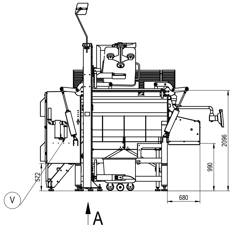
SCHNITT B-B
